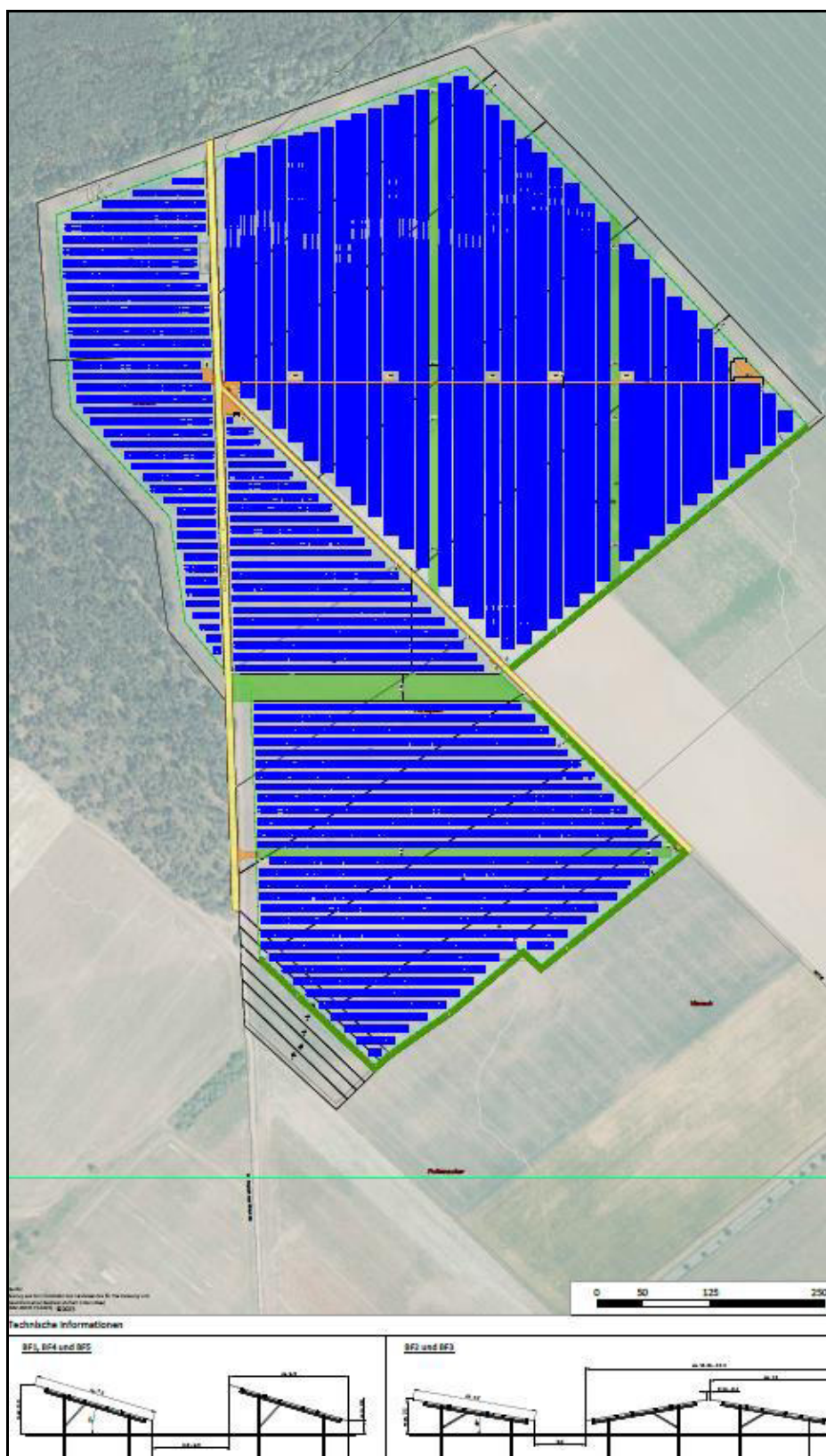
Abbildung 2: Vorhaben- und Erschließungsplan
